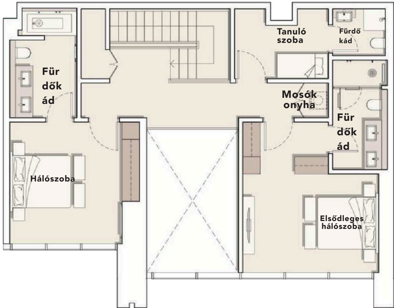
FELSŐ SZINT
